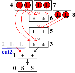
(d) Subgraph 2
